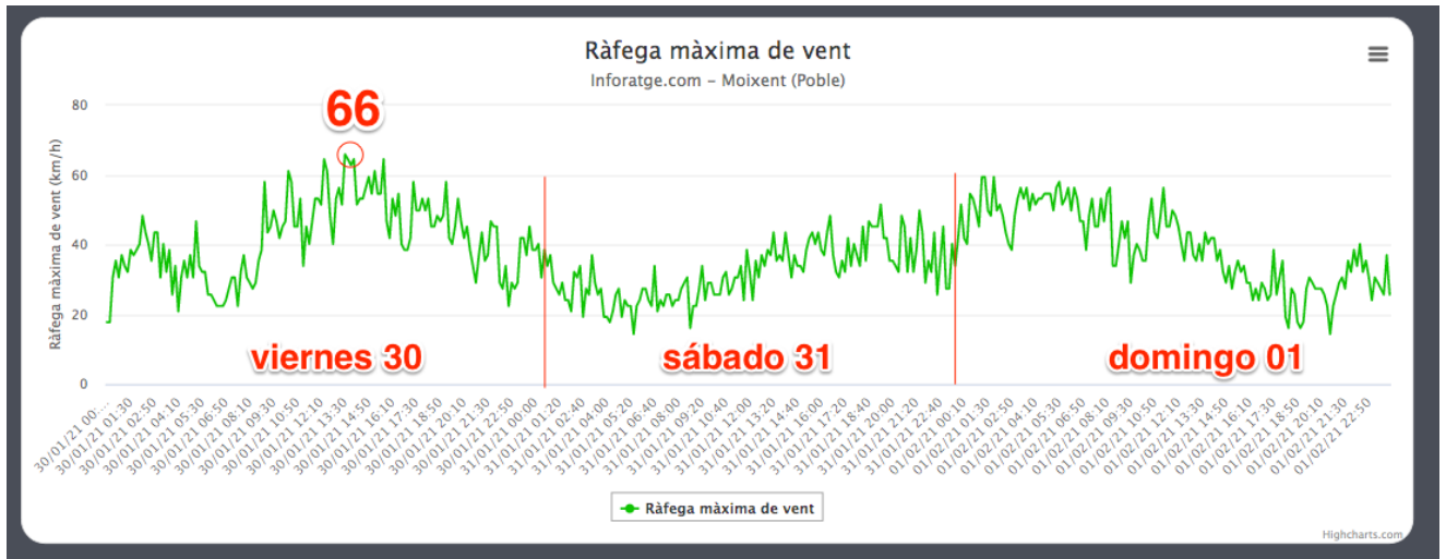
Ráfagas de viento registradas en MOIXENT (poble) entre el 30/01/21 y el 01/02/21 (en km/h) https://inforatge.com/meteo-moixent
