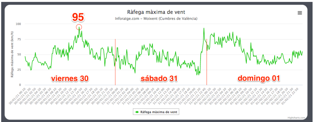
Ráfagas de viento registradas en MOIXENT (Cumbres de València) entre el 30/01/21 y el 01/02/21 (en km/h) https://inforatge.com/meteo-moixent
